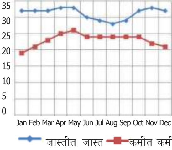
ग्राफ. 2 (सरासरी पणजीतील महिण्याचे तापमान)
