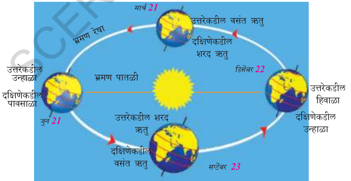
चित्र 3.3 सुर्य, पृथ्वी आणि ऋतु
